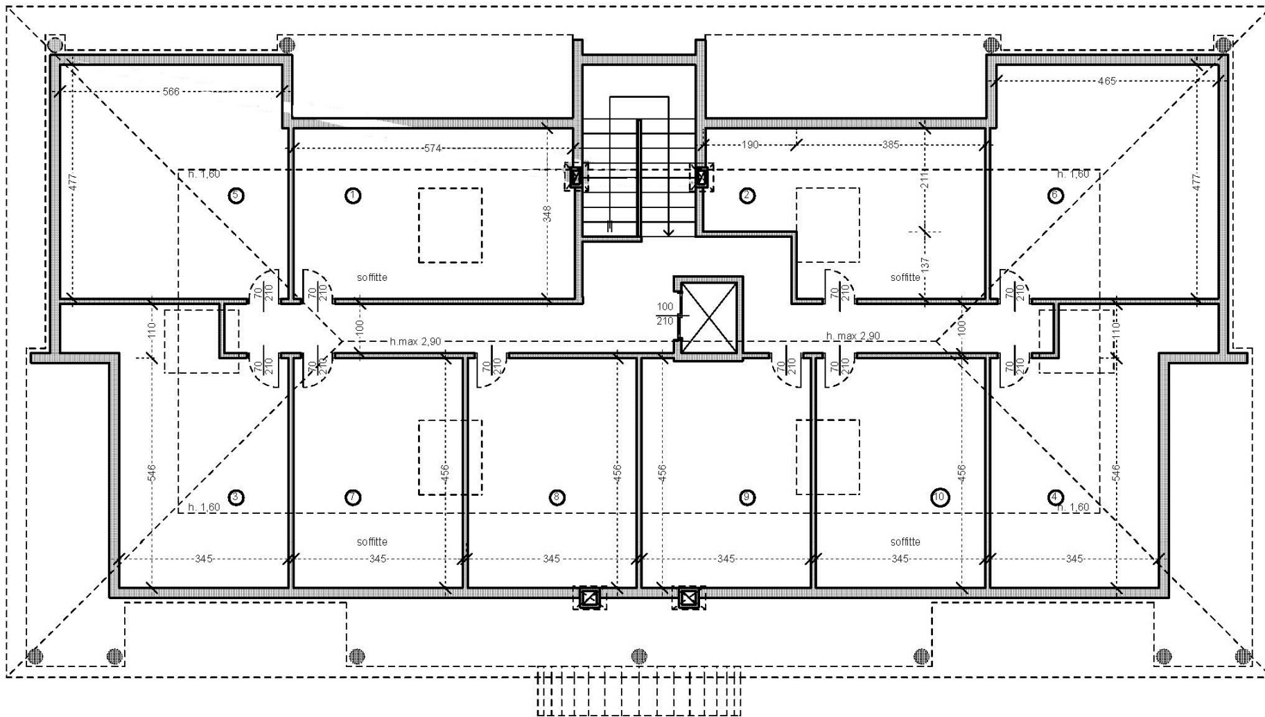
RIPOSTIGLI SOTTOTETTO
